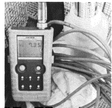
写真3 水質モニタリング機器（W-22XD）
