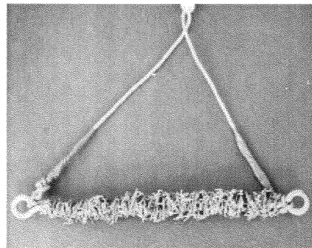
写真2 沈水植物（水草）採集器具
